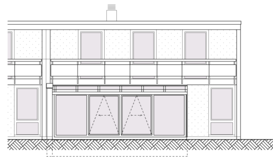
Südwestfassade
