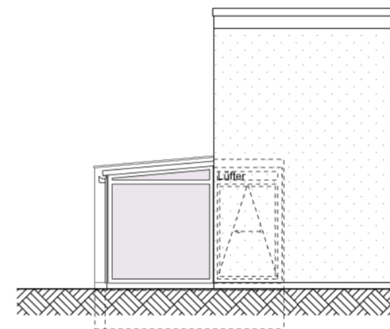
Südfassade
