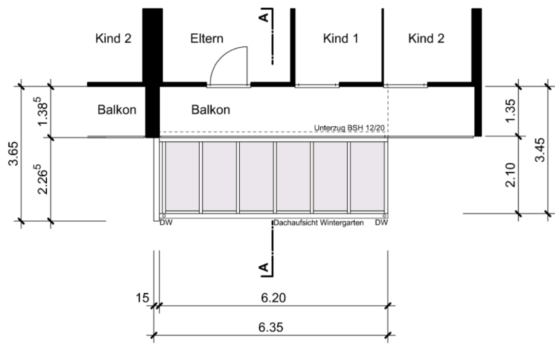
Grundriss Obergeschoss
