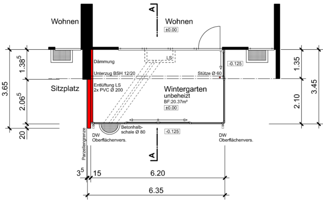
Grundriss Erdgeschoss
