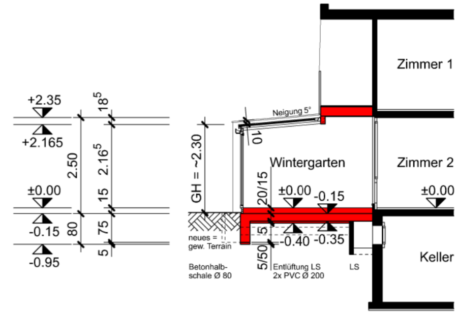
Schnitt A-A
